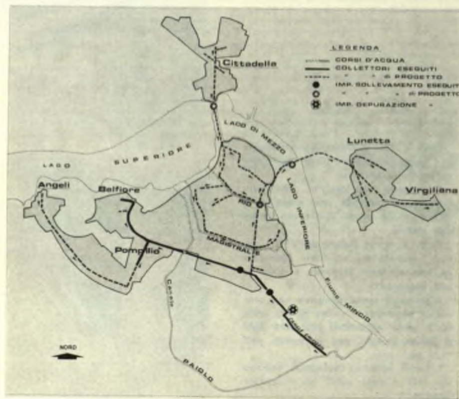
Qui e nella pagina precedente, alcune immagini colte durante l'esecuzione del primo tronco. Sotto, riproduzione della planimetria generale.
