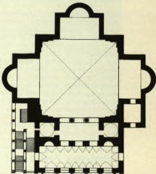
Mantova - L.B. Alberti, San Sebastiano, pianta.
